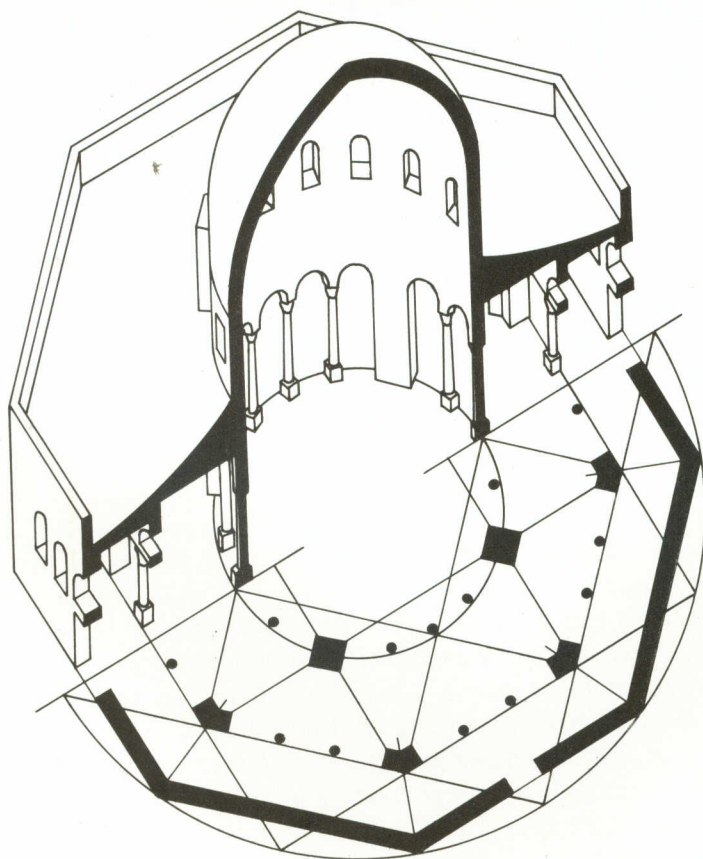
Przekrój aksonometryczny meczetu Umara w Jerozolimie.
